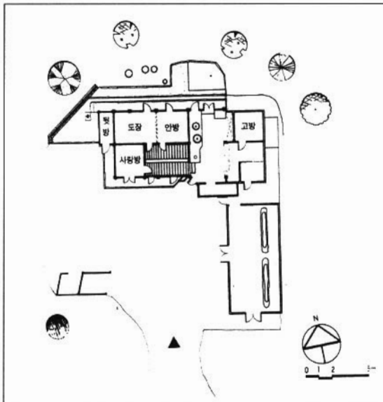
<그림> 장사동 최원규 가옥 평면도
