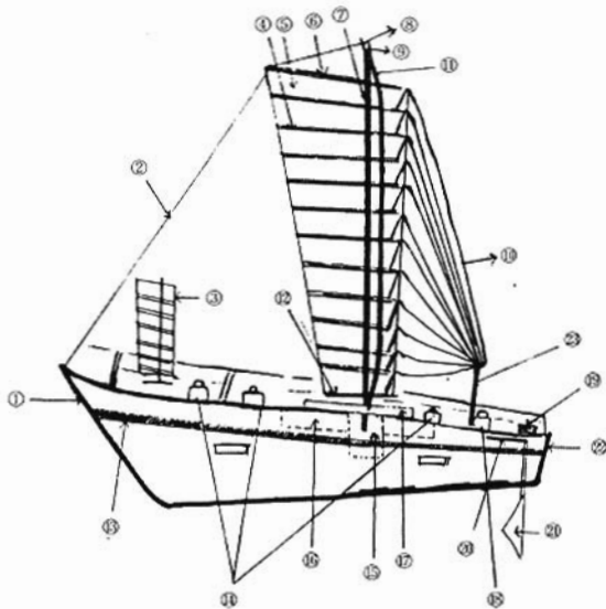
[도표] 돛배의 각 부위 명칭
